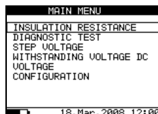
Fig. 5. Main Menu
